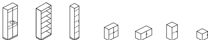
Z7 80x42x205H Z13 80x40x205H Z8 40x42x205H Z9 80x42x78H Z10 80x42x39H Z11 40x42x78H Z12 40x42x39H
